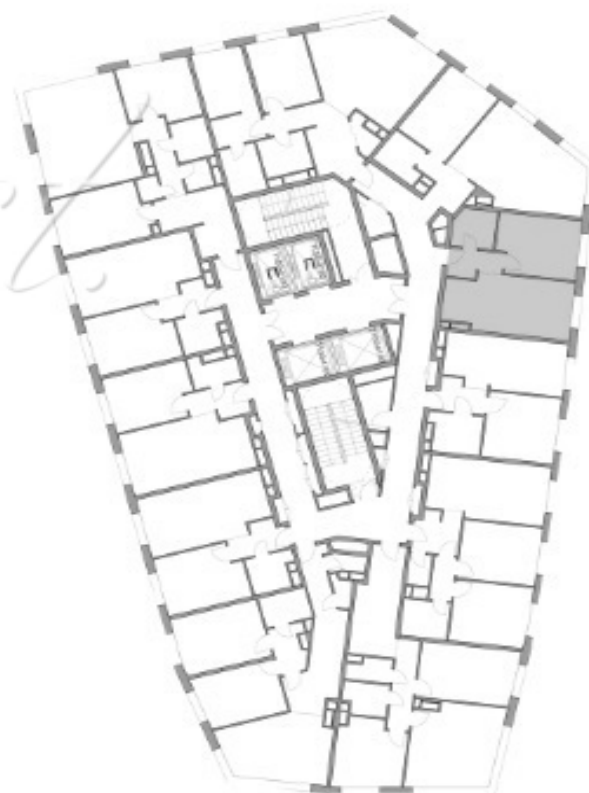
Башня А. План 9-го этажа
